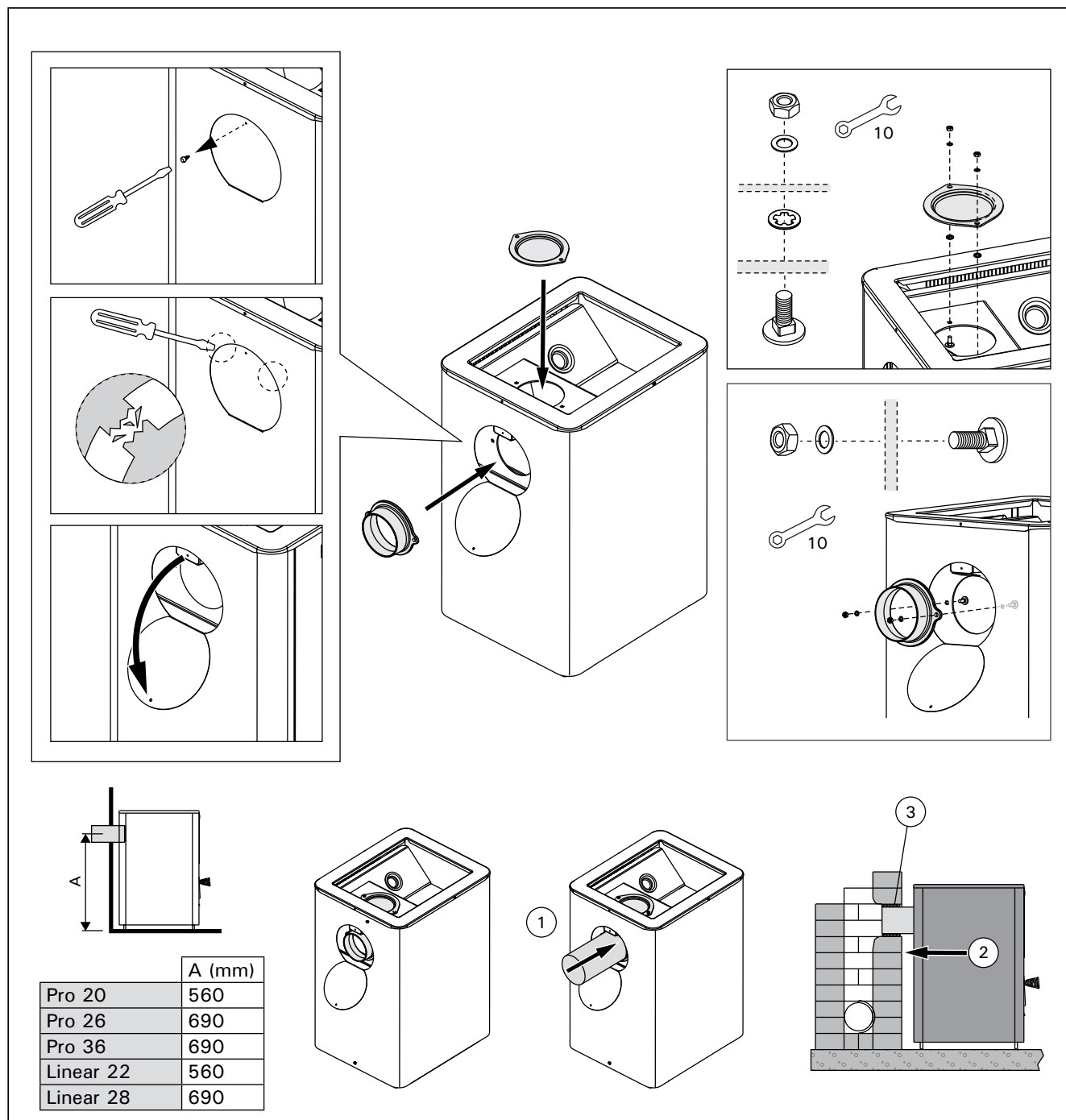
Obrázek 9. Připojení kamen k zděří ve zdi ze zadního otvoru (všechny rozměry jsou uvedené v milimetrech) Figuur 9. De kachel aansluiten op een gemetseld rookkanaal via de aansluitopening achter (alle afmetingen in millimeters)
