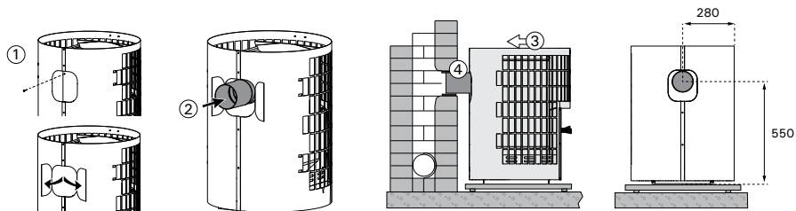
Figuur 9. De saunakachel aansluiten op een gemetseld rookkanaal via de opening aan de achterkant.
